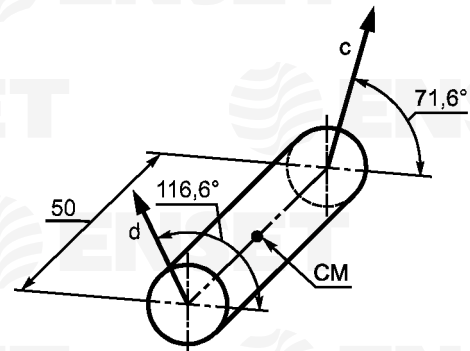
д) Векторы дисбалансов в торцовых плоскостях ротора
