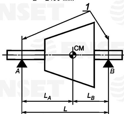
Рисунок А.1 — Геометрические размеры ротора
